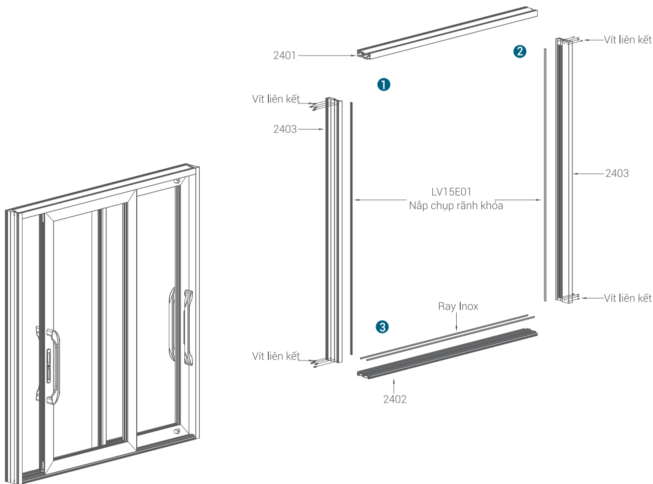
Chi tiết ráp khung bao Outer frame details
